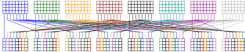
Fig. 4. ShiftColumns of Mysterion-256.
